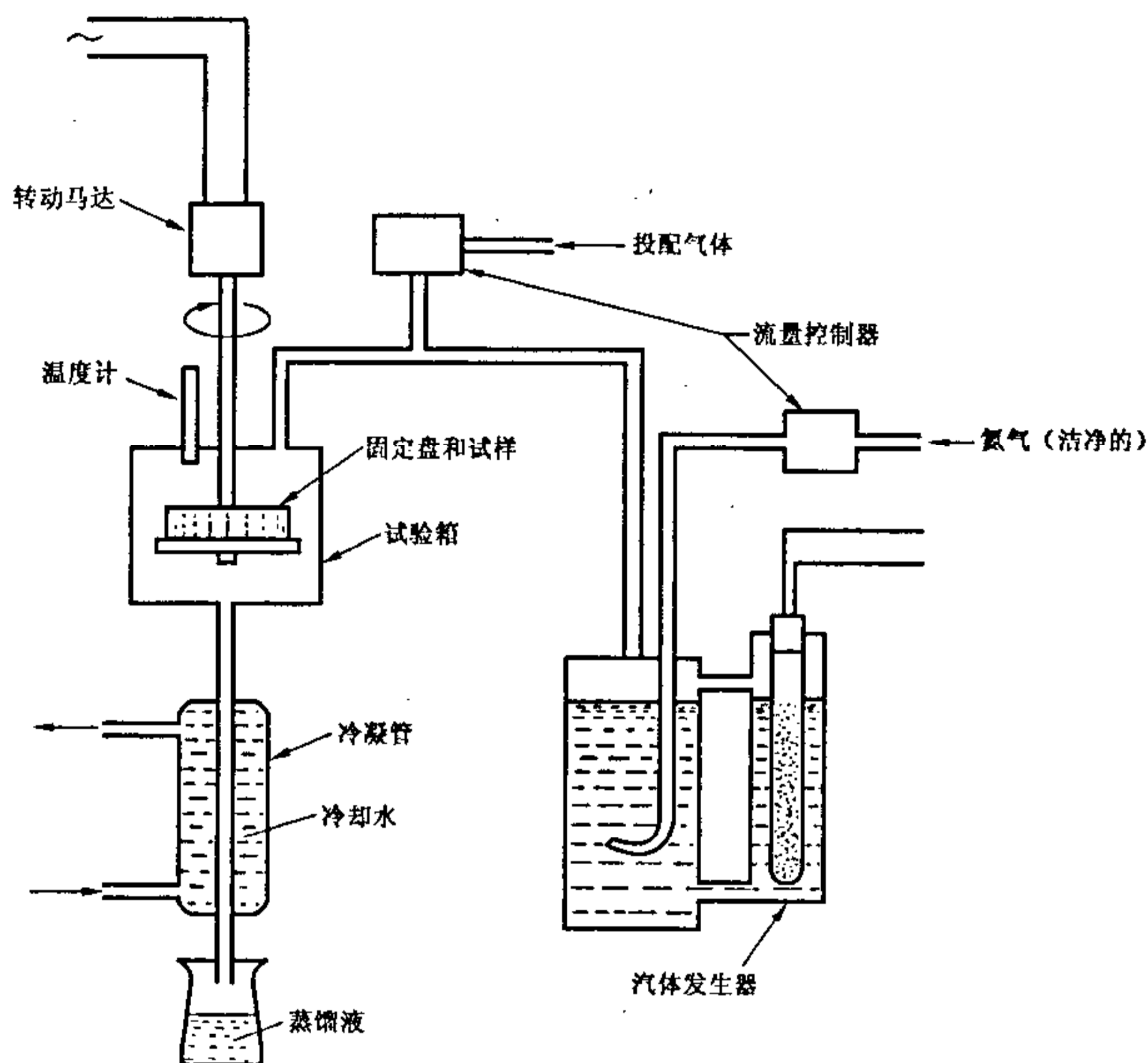
图 18 蒸汽/氧气老化试验设备原理示意图
