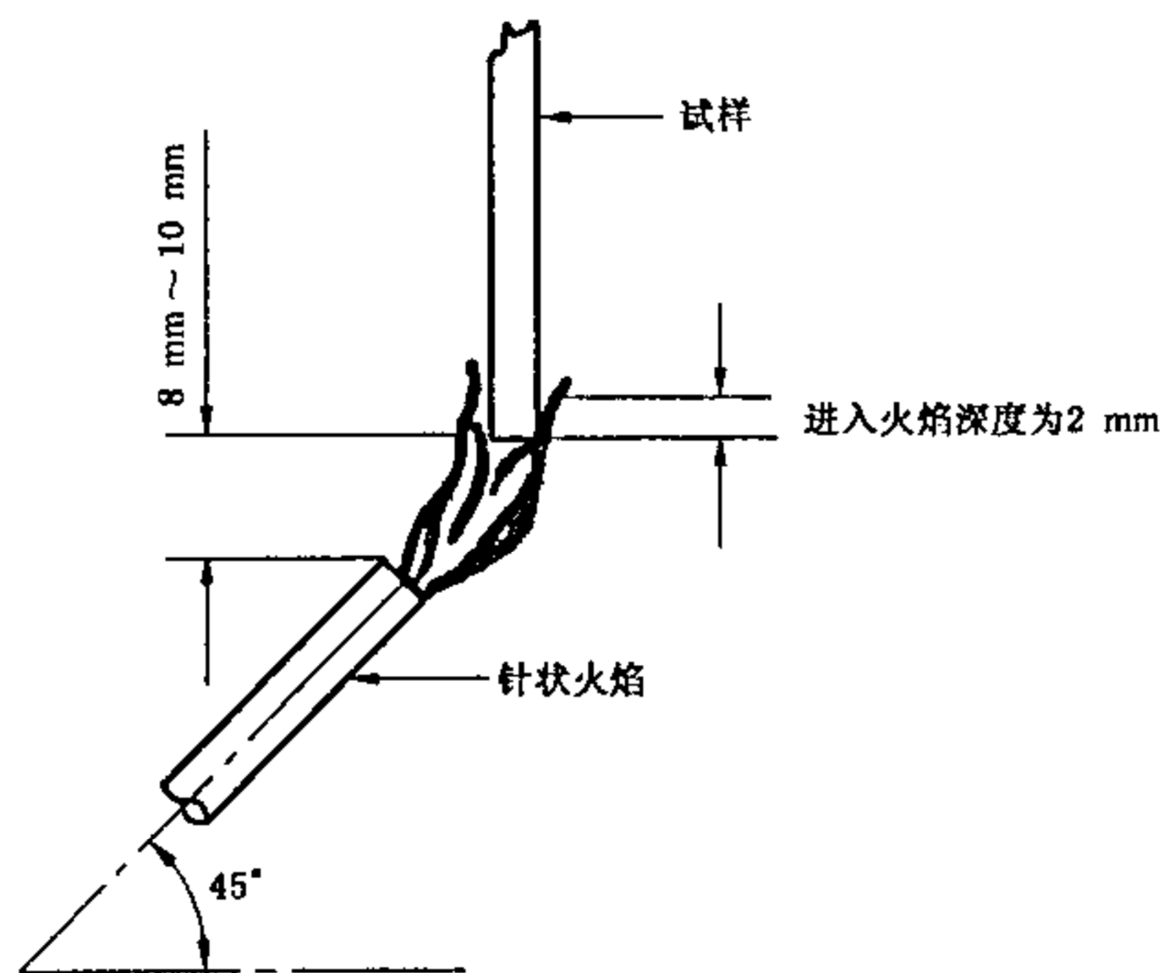
c 试样处于垂直位置
