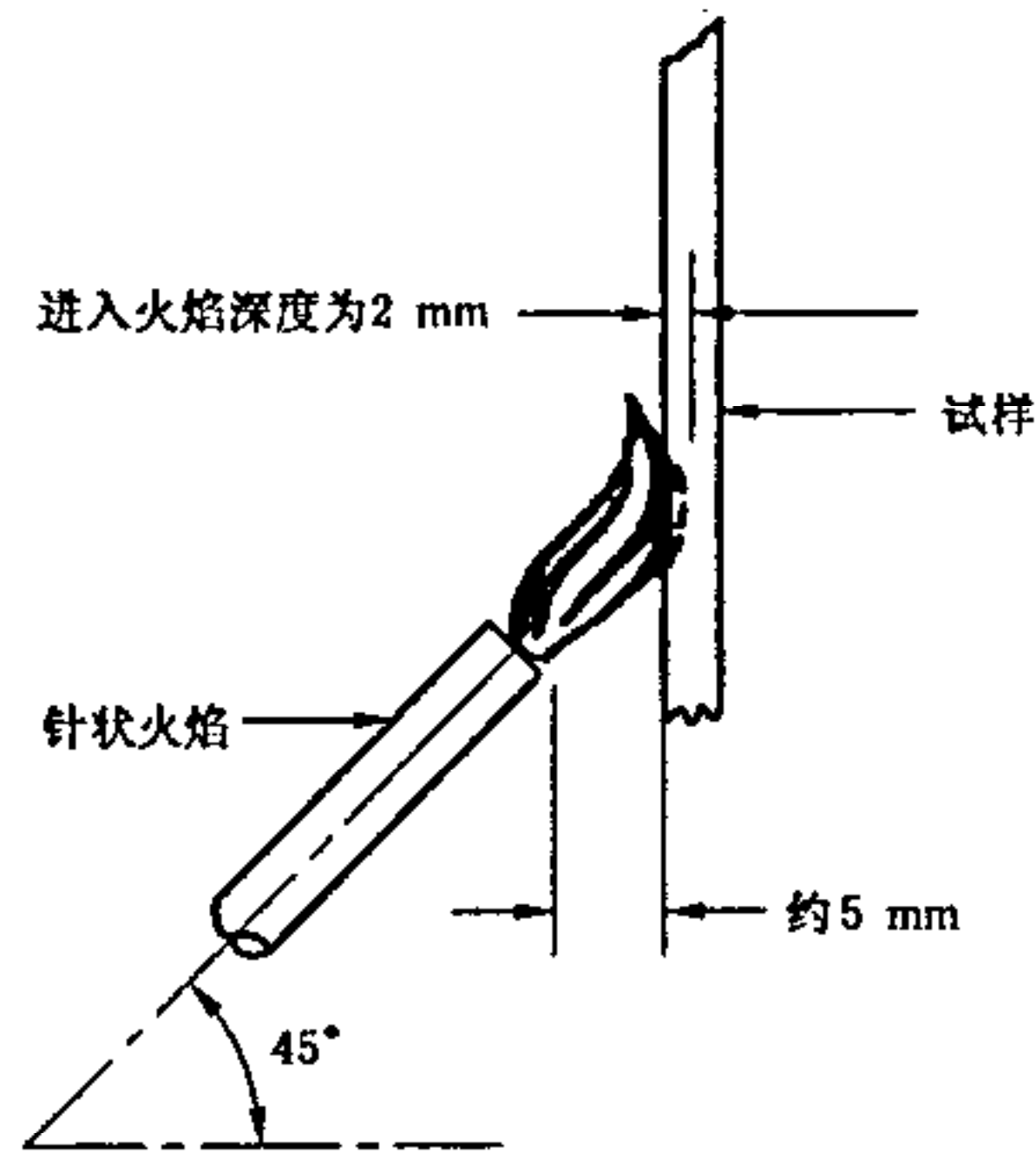
d 试样处于垂直位置
