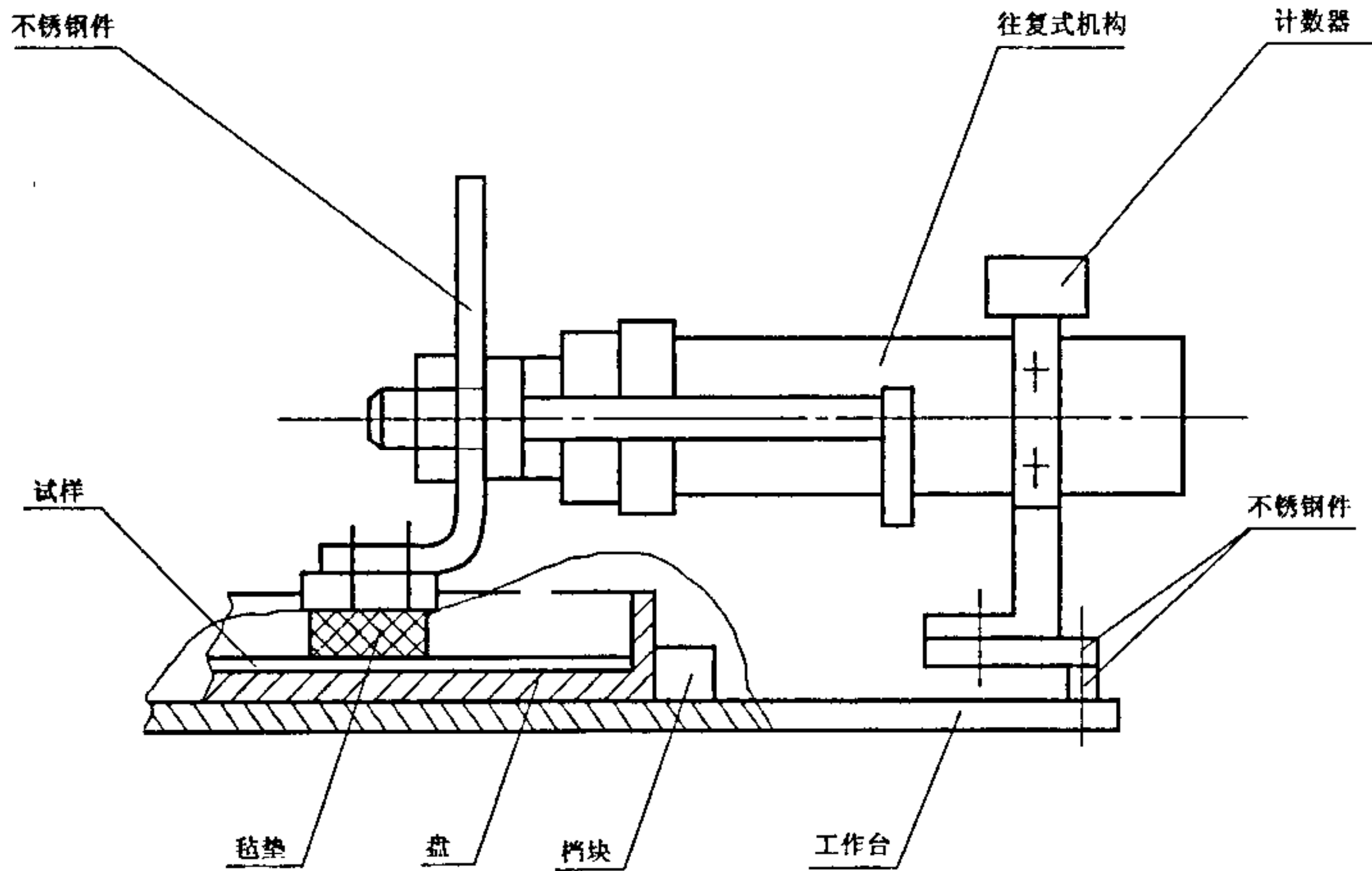
图 13 磨擦试验装置示意图
