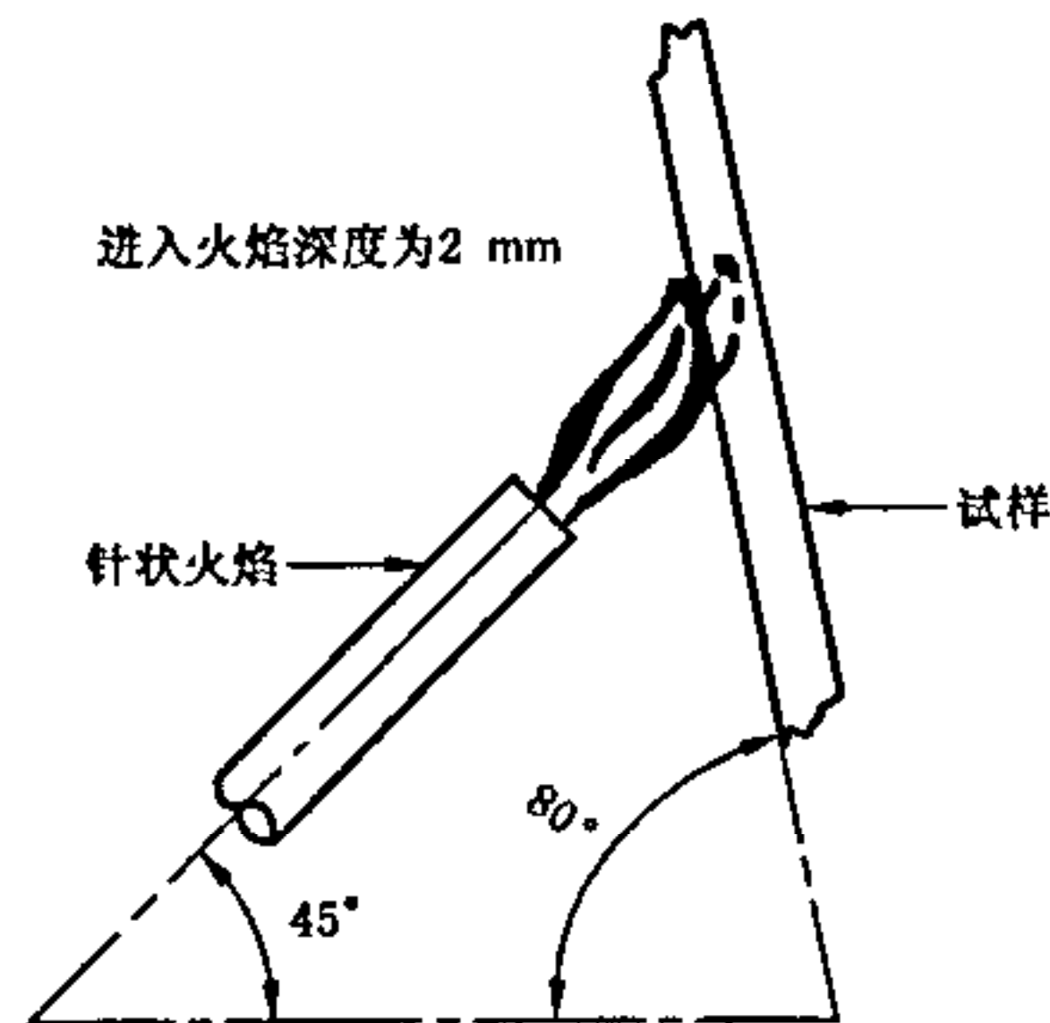
e 试样处于80°倾斜位置
