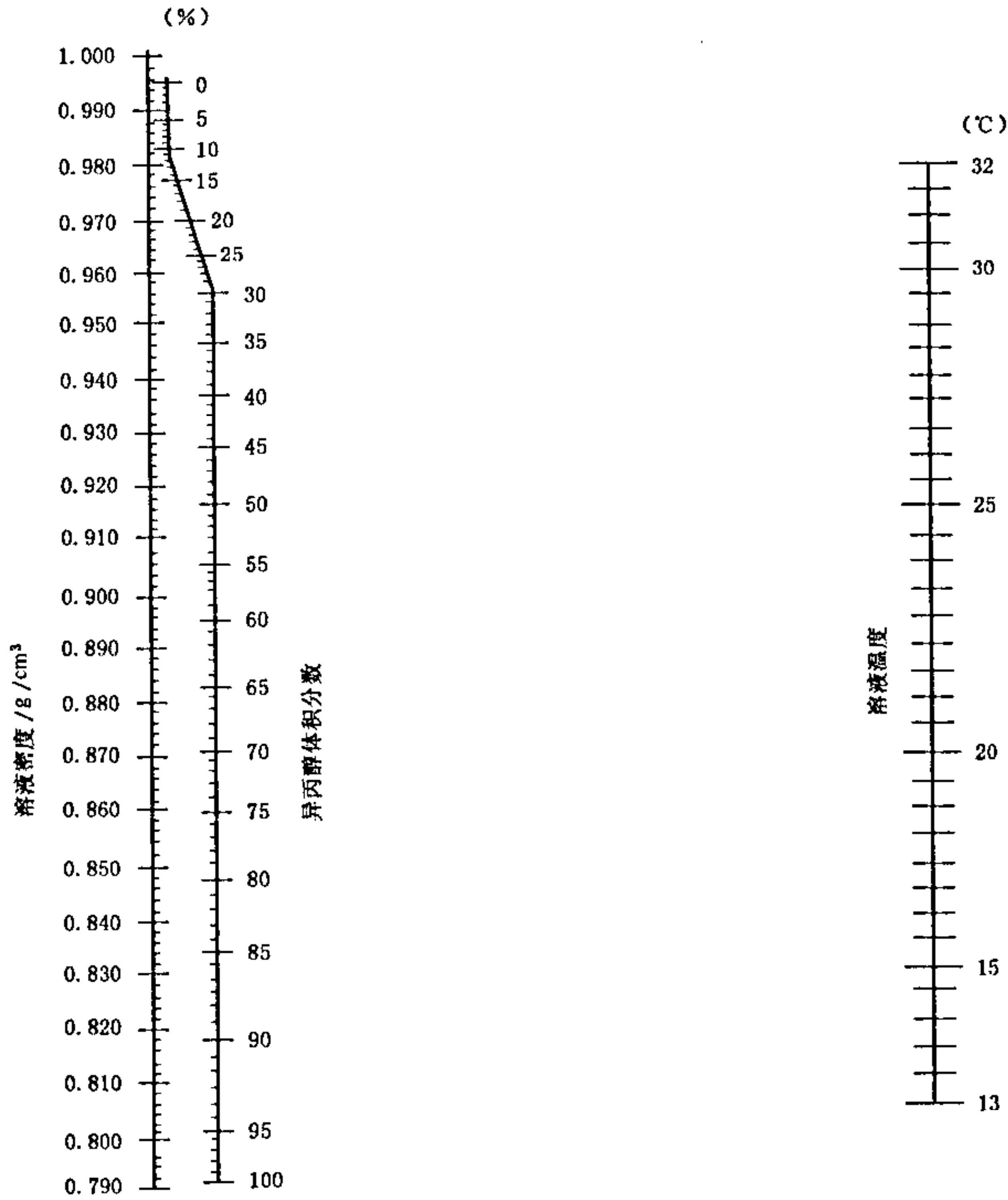
图 19 异丙醇溶液质量浓度计算图解
