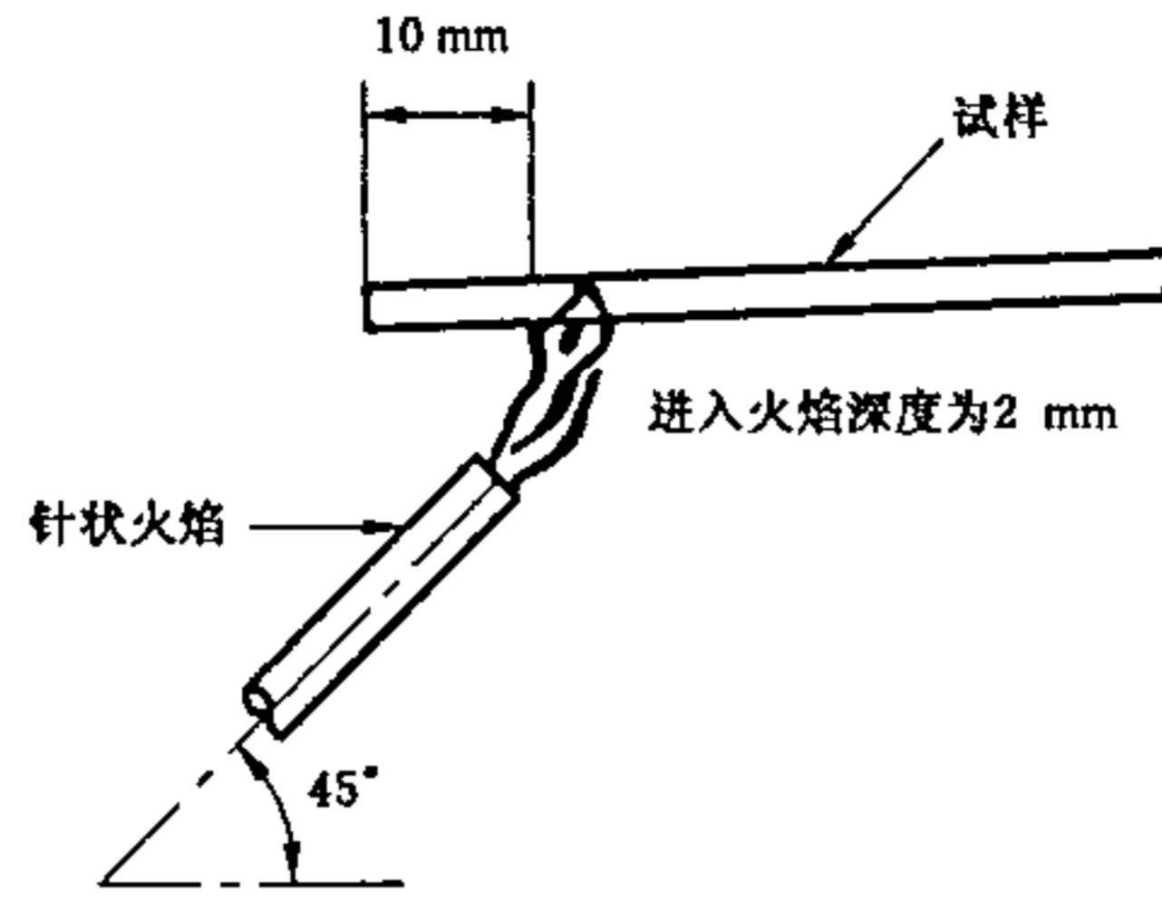
a 火焰施加于表面
