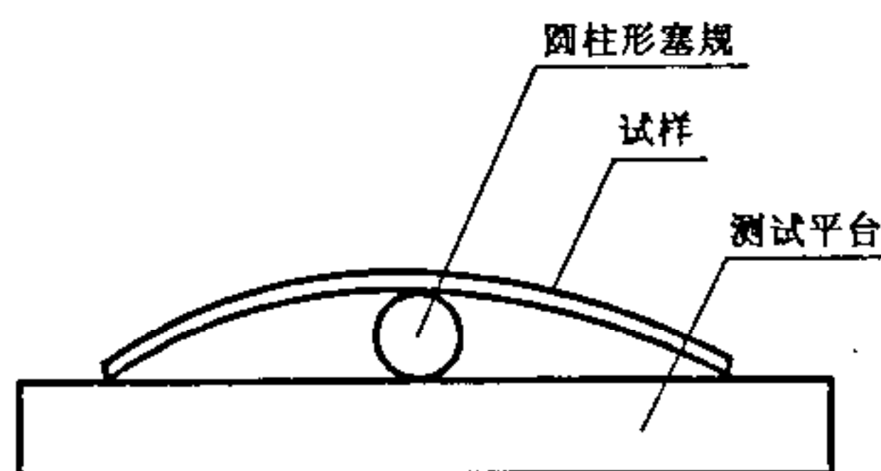
图6 翘曲度塞规法测试示意图
