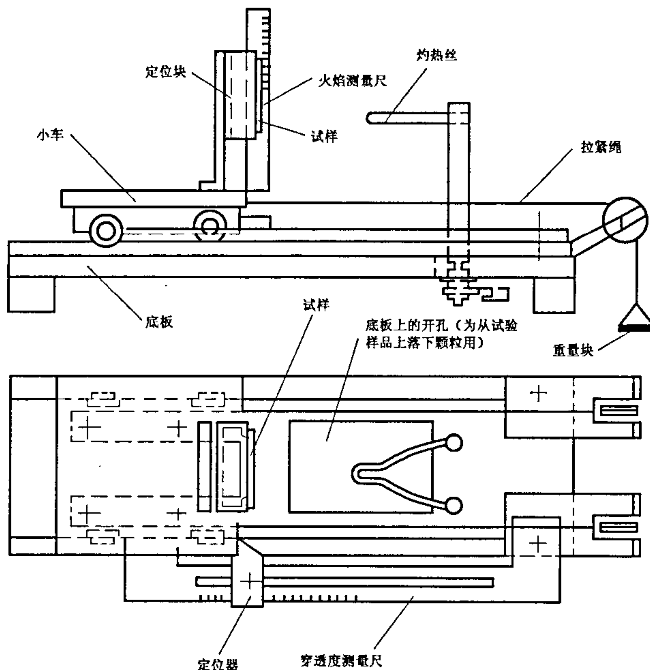
图 11 灼热丝试验装置示意图
