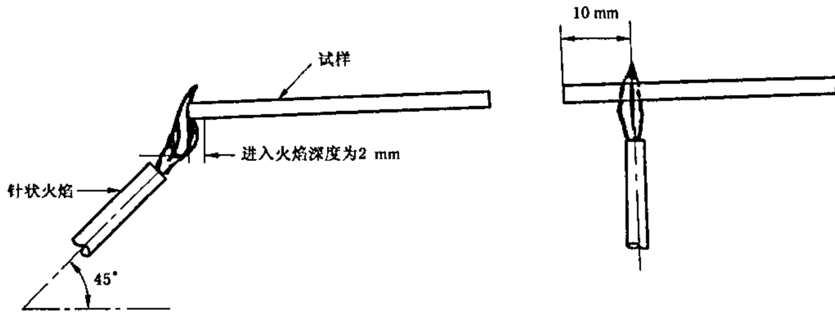
b 试样处于水平位置
