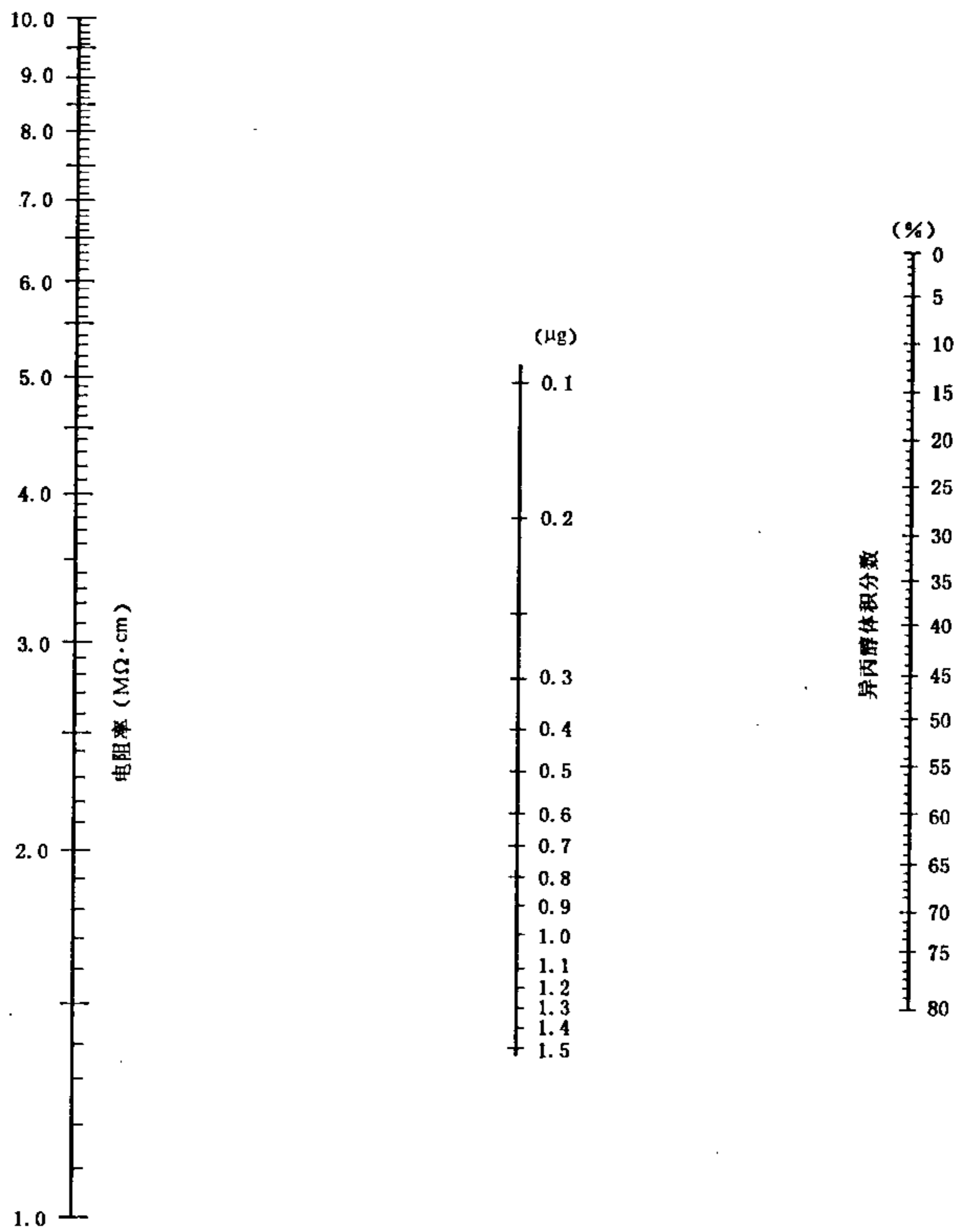
图 20 氯化钠质量浓度计算图解
