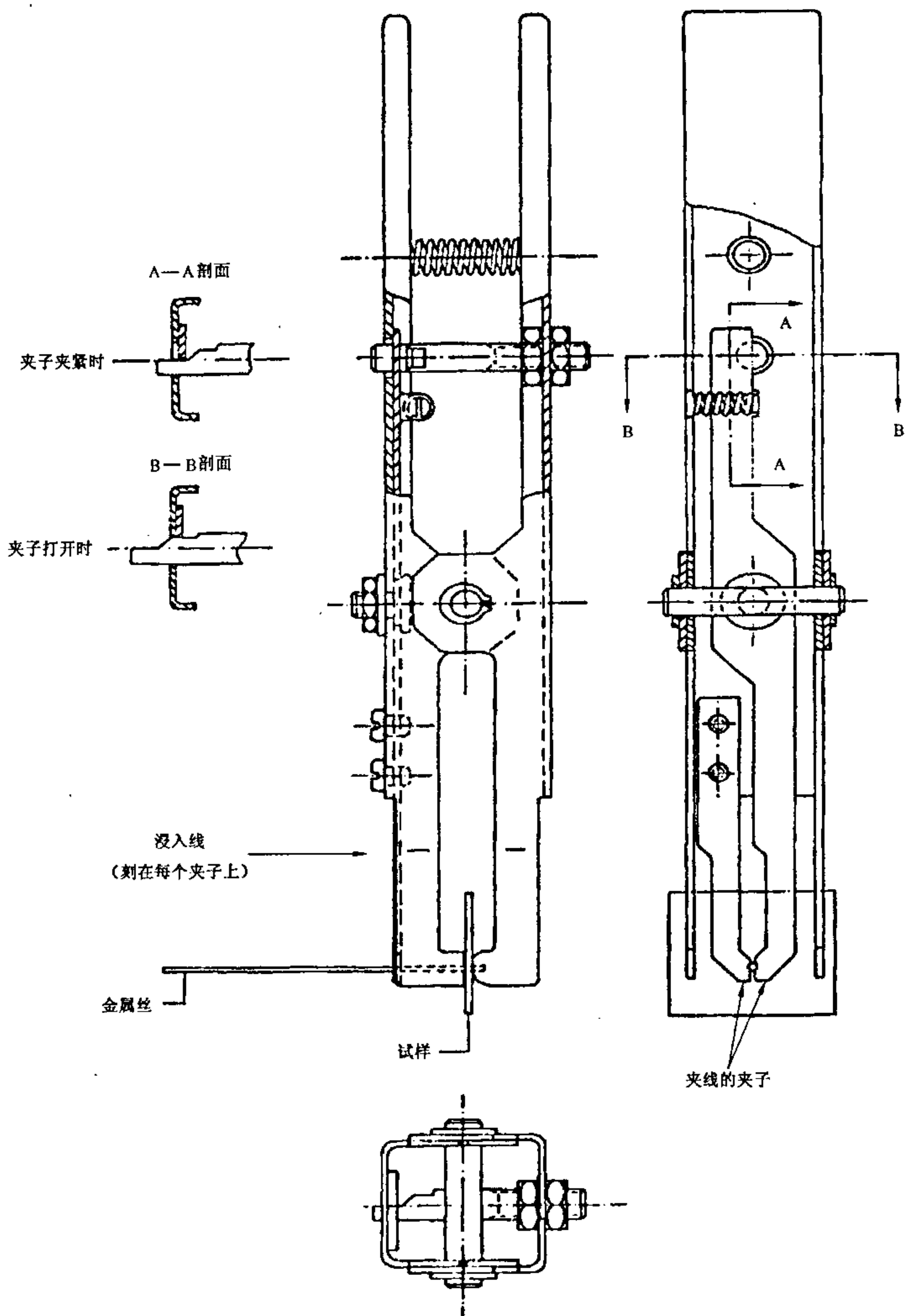
图 16 热应力 浸焊试验用夹具
