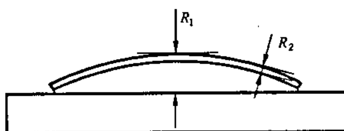
图5 翘曲度计算法测试示意图
