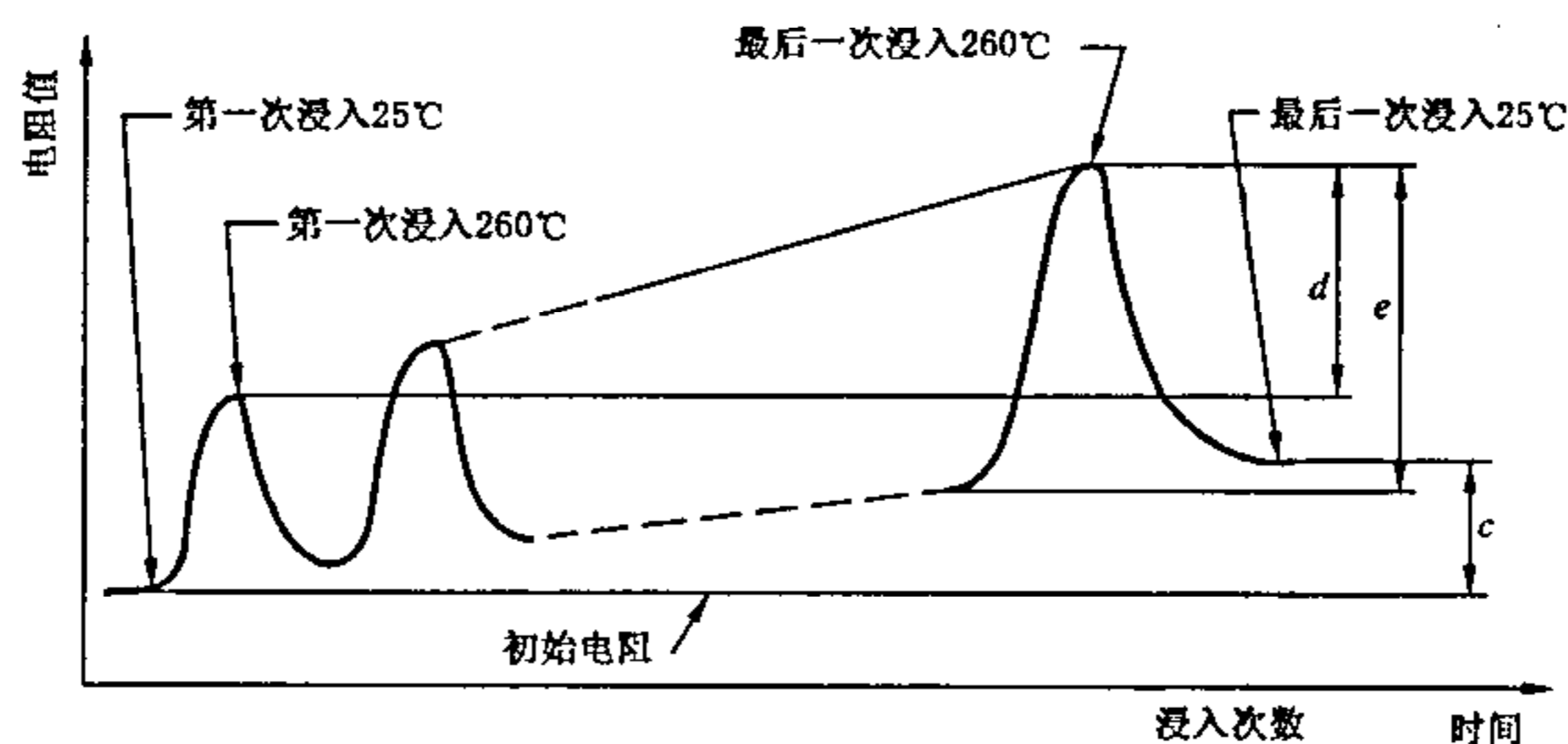
图 4 热循环浸泡次数与电阻值曲线
