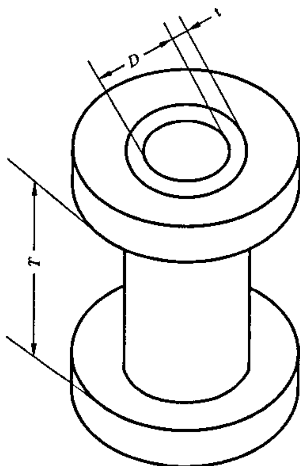
图 8 金属化孔几何尺寸示意图
