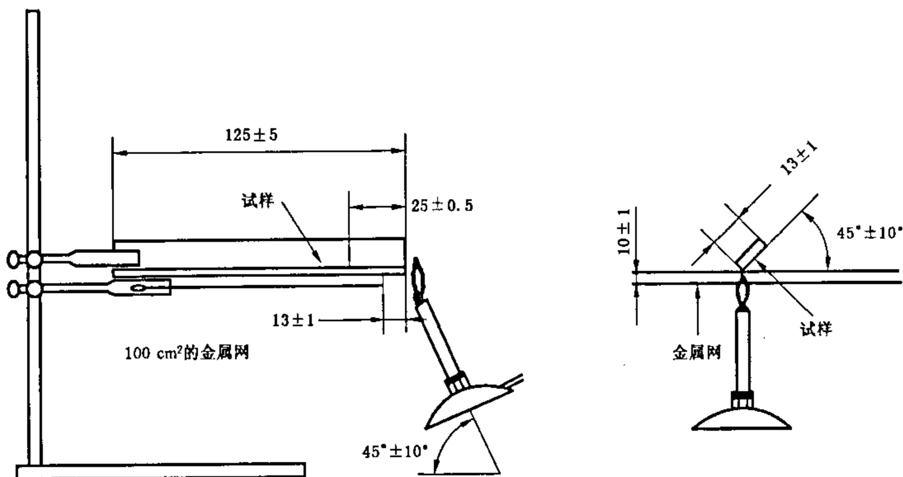
图 10 水平燃烧试验
