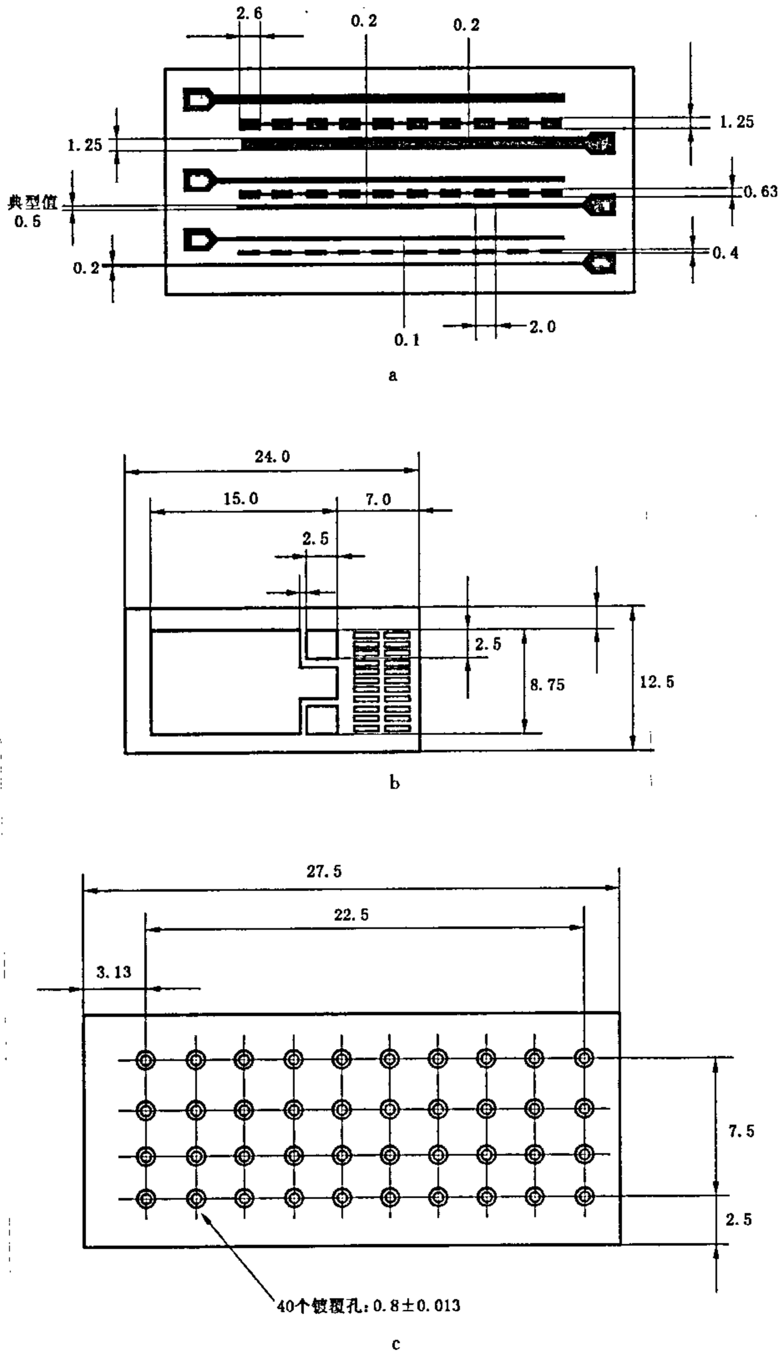
图 17 典型的测试图形
